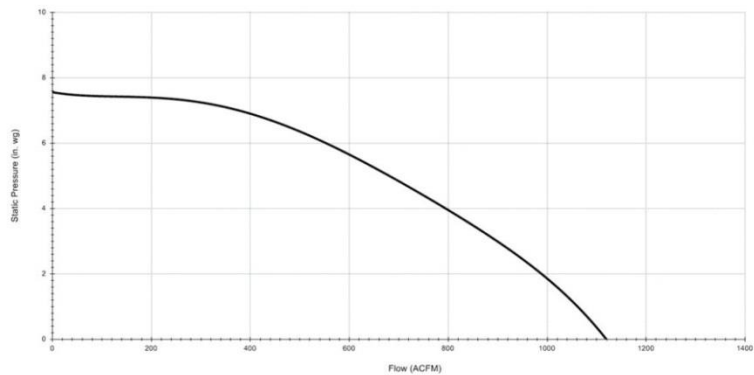
SP-1000LV FAN CURVE
