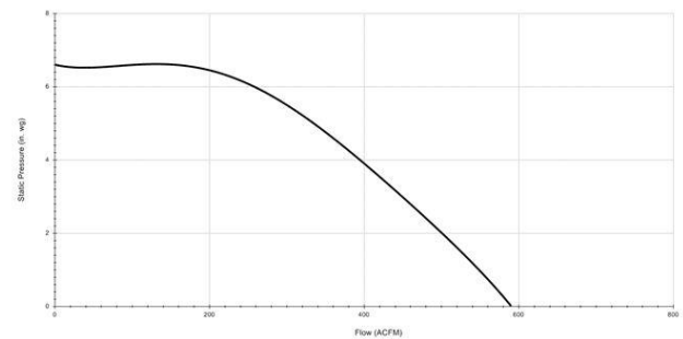
MAC-21 FAN CURVE
