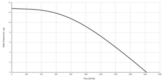
PFB-1600 FAN CURVE
