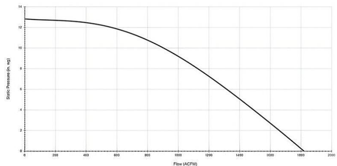
PFB-1600VFD FAN CURVE
