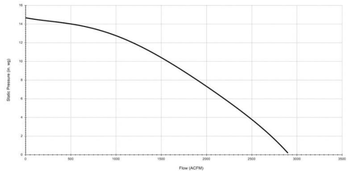
PFB-2500SP FAN CURVE
