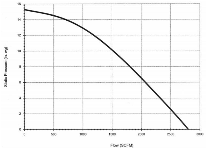
PFB(H)-2500A Fan Curve
