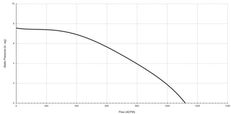
SP-1000LV FAN CURVE
