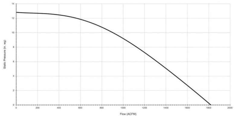
SP-1600 FAN CURVE
