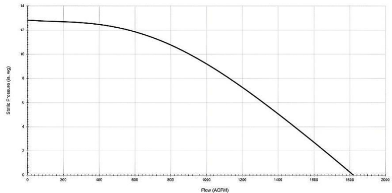
SP-1600VFD FAN CURVE
