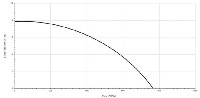
SP-700 FAN CURVE
