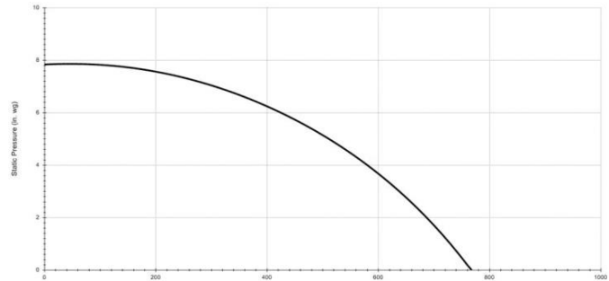
SP-700EP FAN CURVE
